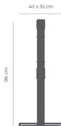
Poste MAX DUAL Esc. 1:20 (Peso: 11Kg)
