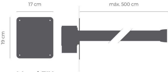
Mural FIX Esc. 1:10 (Peso: 1kg)
