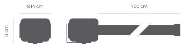
Mural ESTÁNDAR 7m
