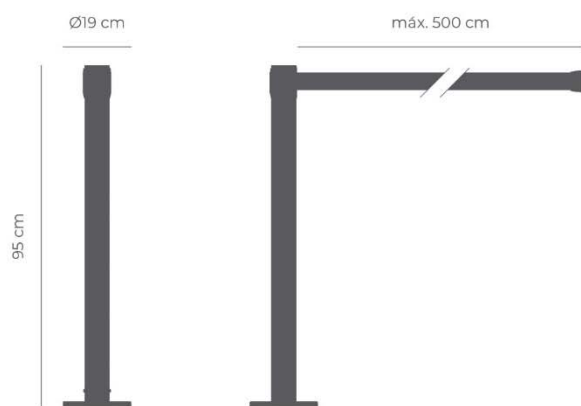
Poste FIX Esc. 1:20 (Peso: 4kg)
