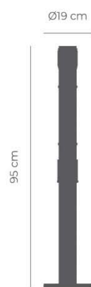
Poste FIX DUAL Esc. 1:20 (Peso: 4Kg)
