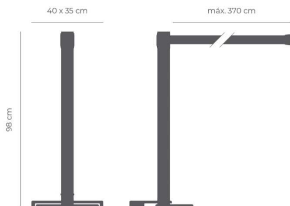
Poste MAX Esc. 1:20 (Peso: 11kg)
