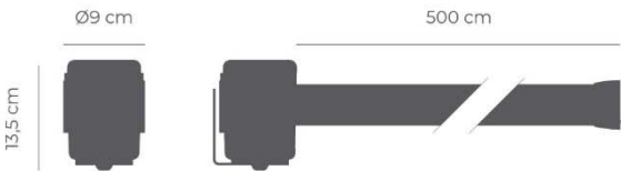
Mural ESTÁNDAR 5m Esc. 1:10 (Peso: 1kg)
