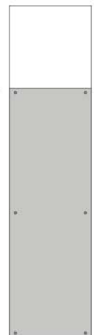
sil 206 VV SS w 270 x h 1080 x d 14mm w 10,63 x h 42,52 x d 0,55"
